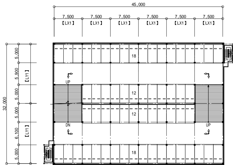
1階 平面図
